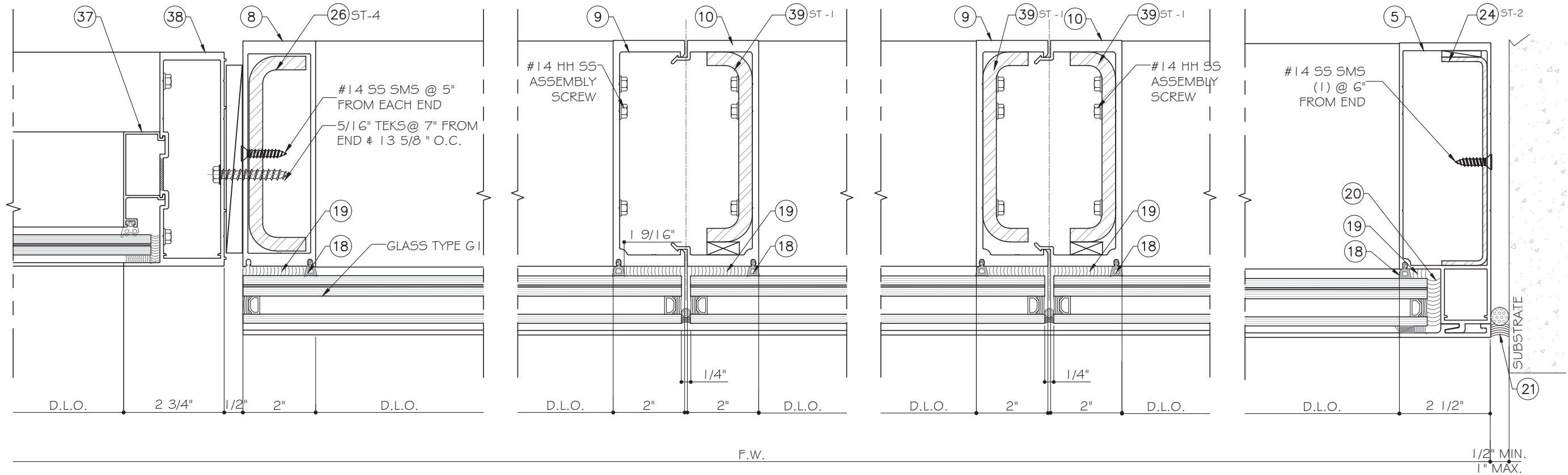
11 D3 DETAIL
